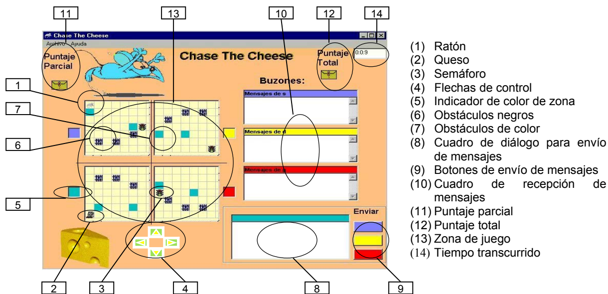
Figura 1. Componentes de la interfaz gráfica de Chase the cheese .
